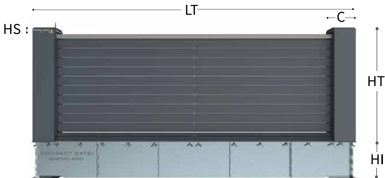
VISTA FRONTALE - Front view - Frontalansicht - Vista frontal - Vue de face
